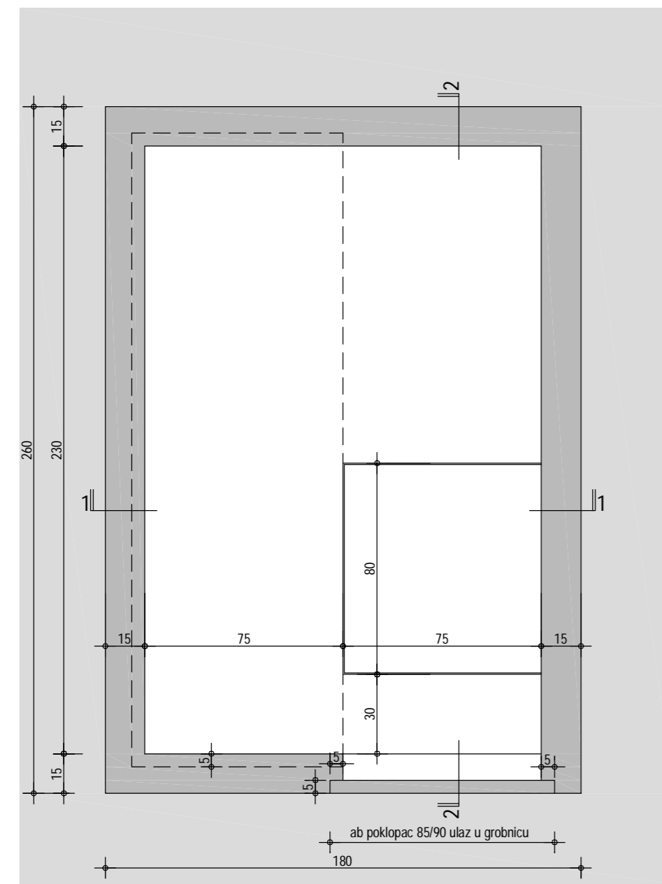
TLOCRT
