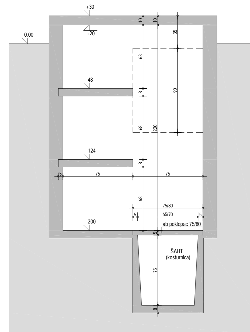
PRESJEK 1-1
