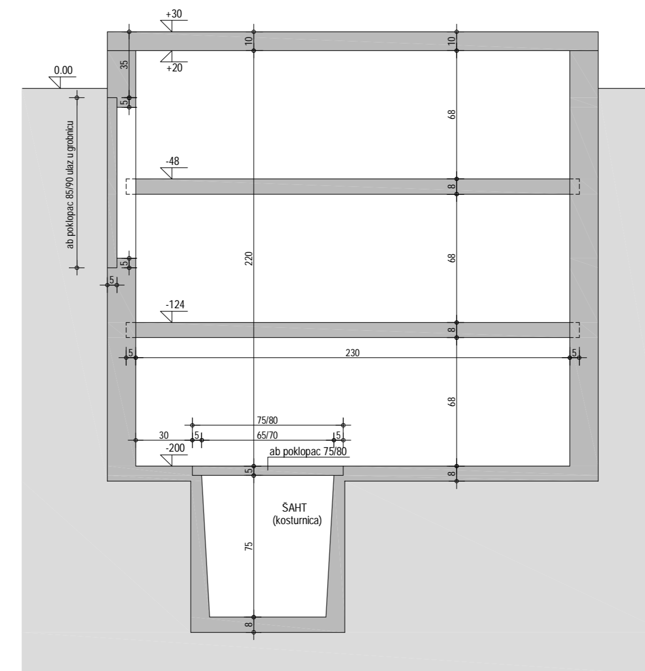
PRESJEK 2-2
