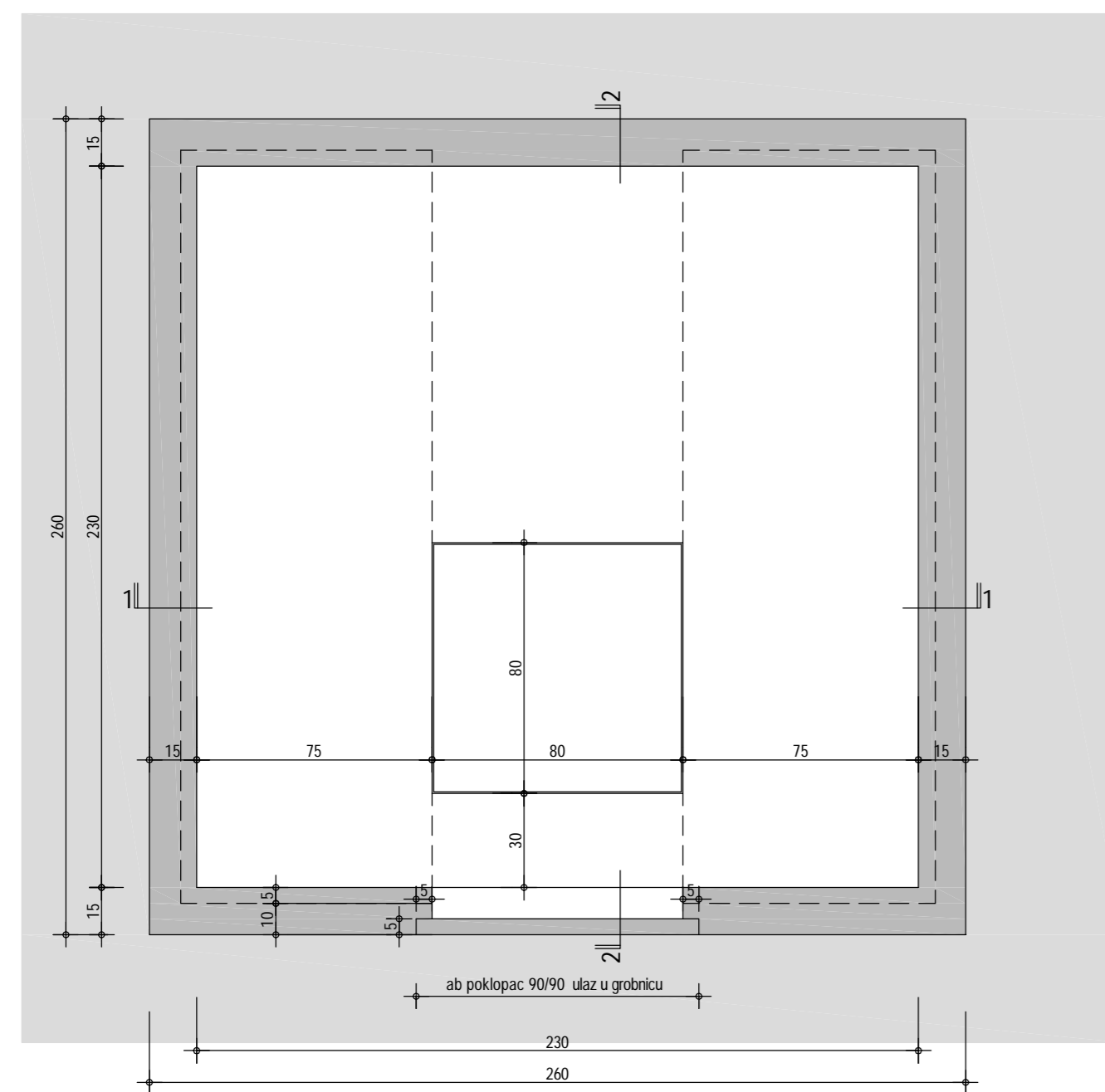
TLOCRT
