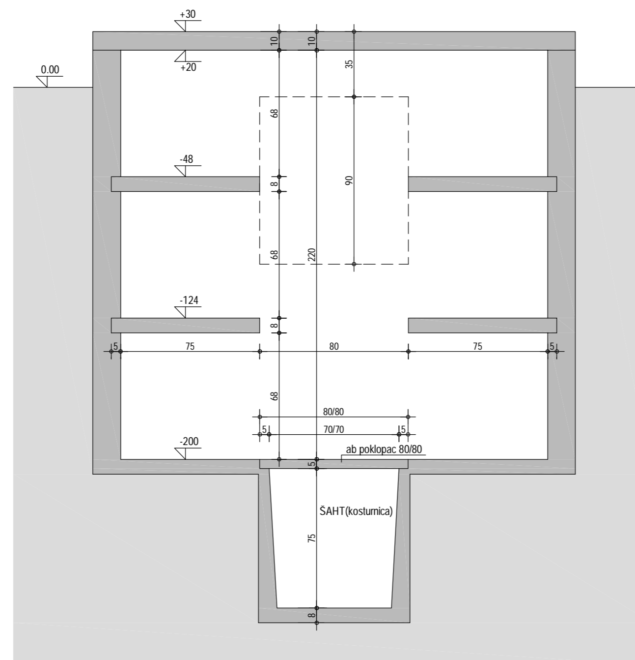
PRESJEK 1-1
