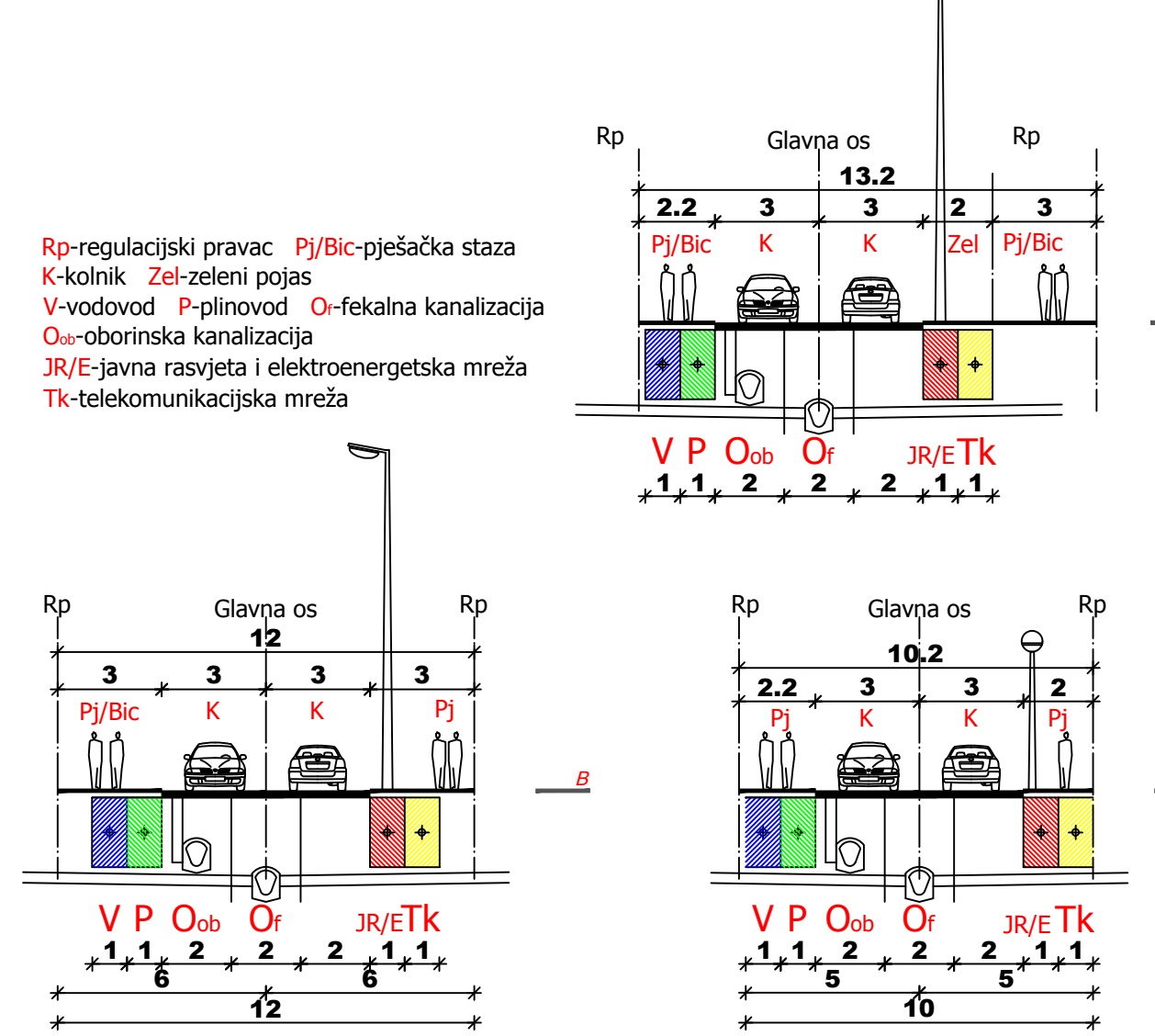
KARAKTERISTIČNI POPREČNI PRESJECI ULICA - m.1:200
